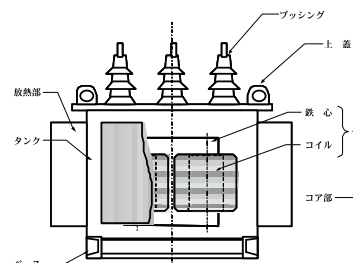
高压変圧器の例
